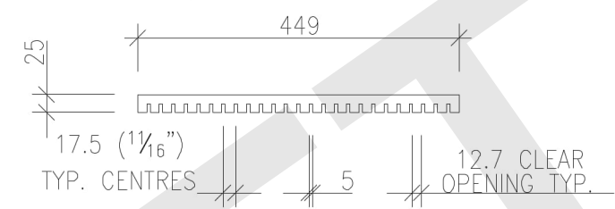
SPACER BAR 'A'
