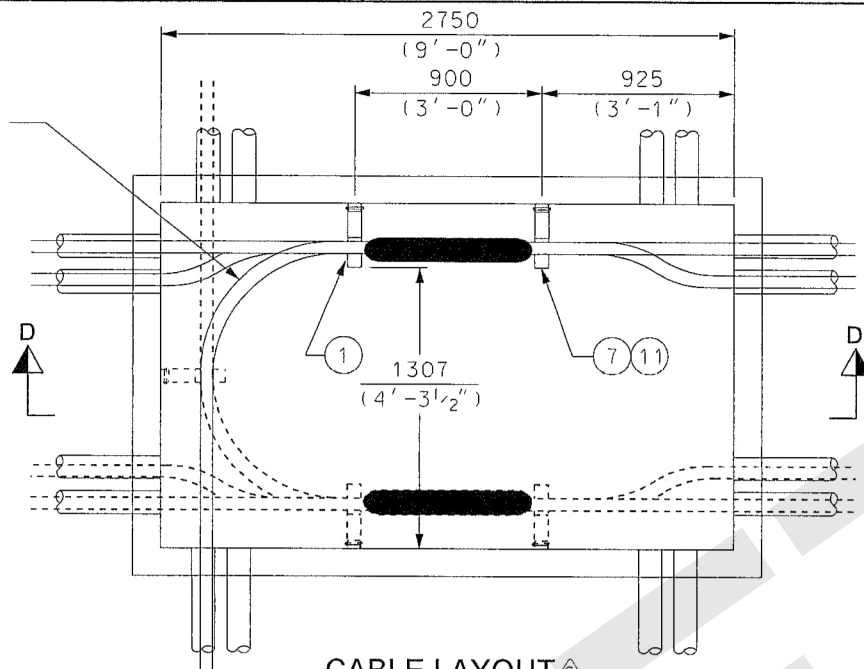
CABLE LAYOUT Ⓐ
