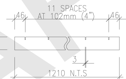
LOAD BAR 'B'
